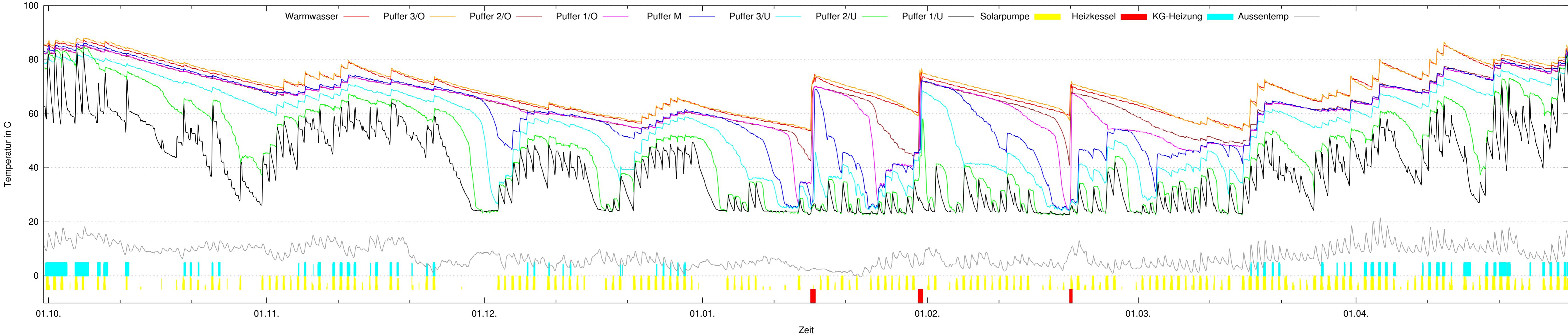
Solarwerte Winterhalbjahr 2015/2016
