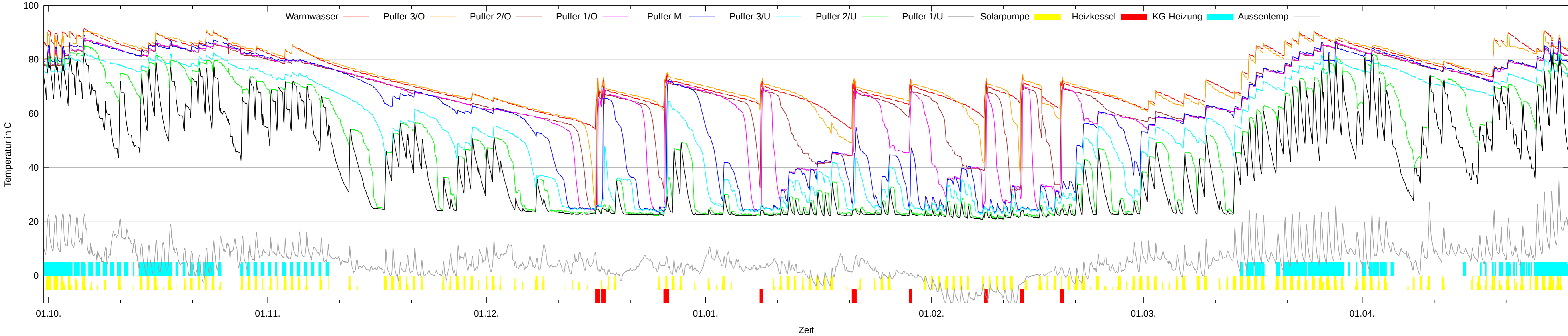
Solarwerte Winterhalbjahr 2011/12
